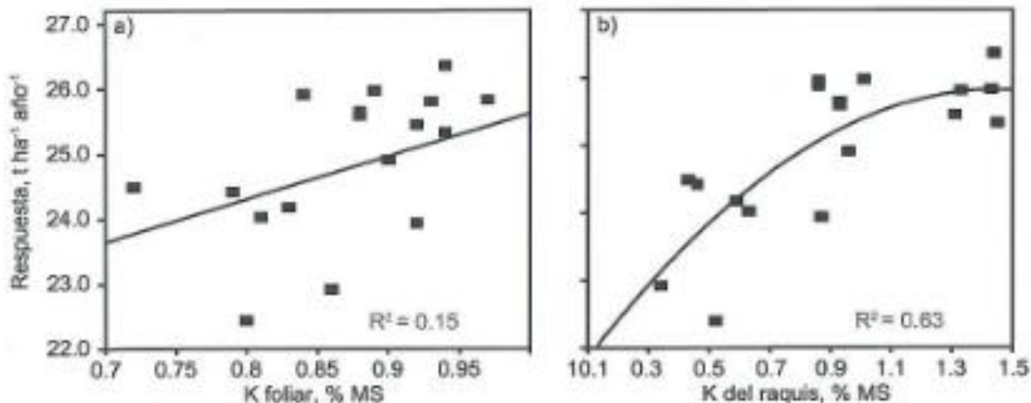
Figura 14. Comparación de la relación entre el rendimiento y la concentración de K foliar (a) y tejido del raquis (b) en un experimento de fertilización en suelo volcánico en el Norte de Sumatra (Foster y Prabowo, 1996a).
