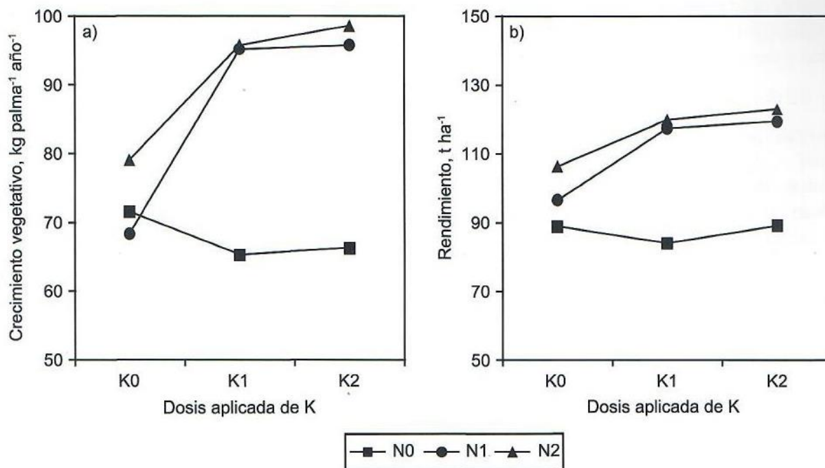
Figura 12. Efecto de los fertilizantes de N y K en el crecimiento vegetativo y rendimiento en palmas de aceite en un suelo de la serie Rengam (Typic Paleudult) en Malasia (Chan, 1982a).
